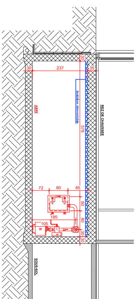
COUPE B-B
