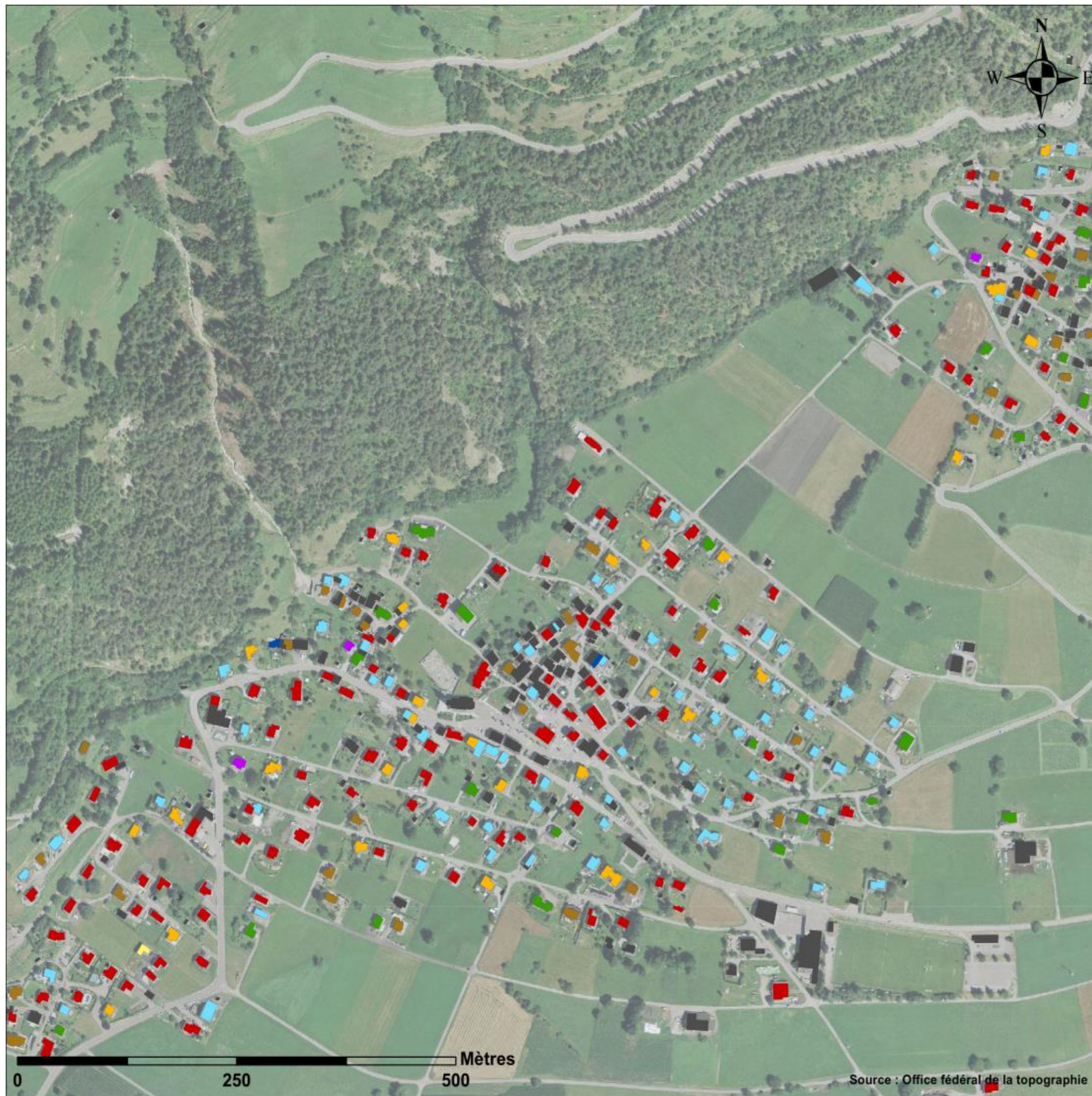
Besoins de chauffage des bâtiments par agent énergétique principal et nombre de bâtiments associés
