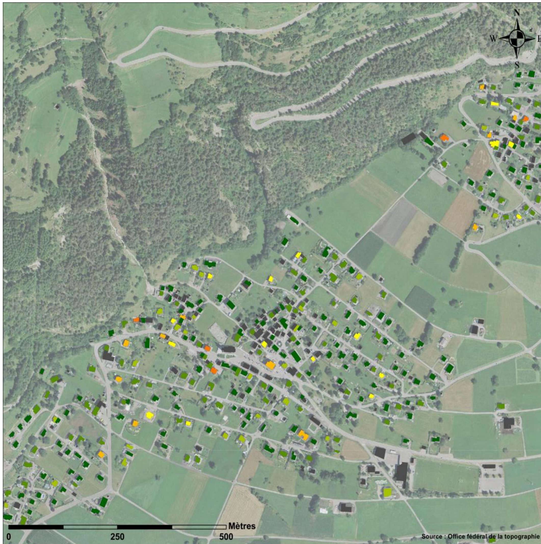
Besoins de chaleur des bâtiments par plage de besoins et nombre de bâtiments associés
