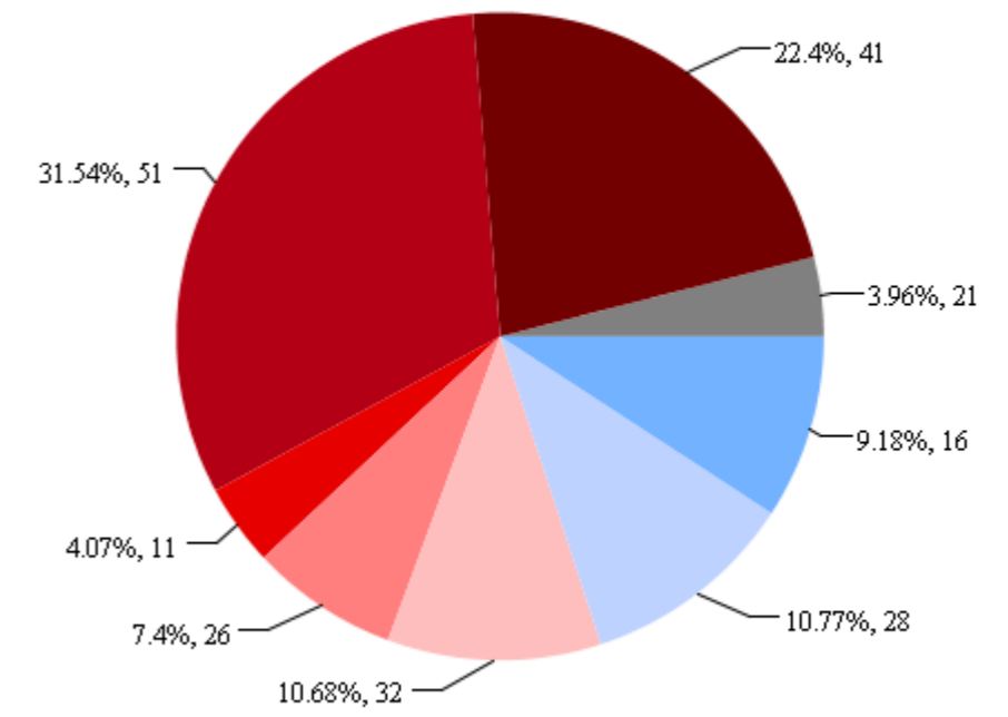
Surface de référence énergétique répartie par époque de référence et nombre de bâtiments associés
