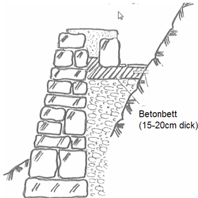
Skizze: WL hinter einer Stützmauer entlang eines Felsens mit Betonbett
