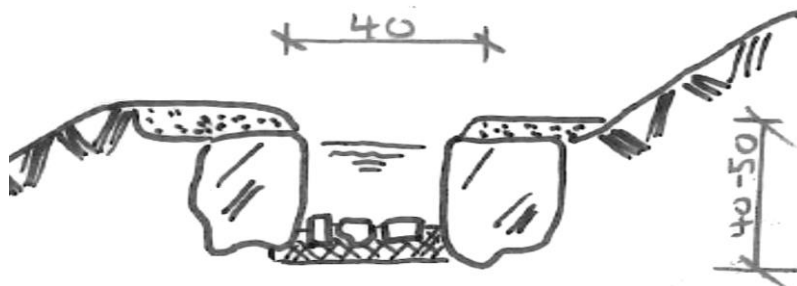
Sohle einer WL mittels einer Sohlenbikki, welche in Mörtel verlegt wird Coupe: lit de bisse consolidé avec des pierres (Sohlenbikki), posée sur un lit de mortier
