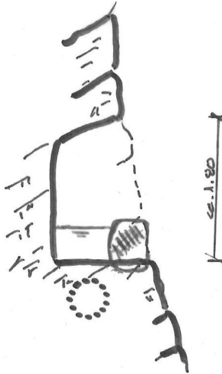
Skizze: Halbgalerie mit Tretschbord / Verrohrung Coupe: demi galerie avec consolidation de la berge droite avec des pierres (Tretschbord) / mise sous tuyau
