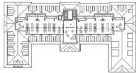
Plan de l'ensemble de l'abbaye de Maya (vue de l'est)
