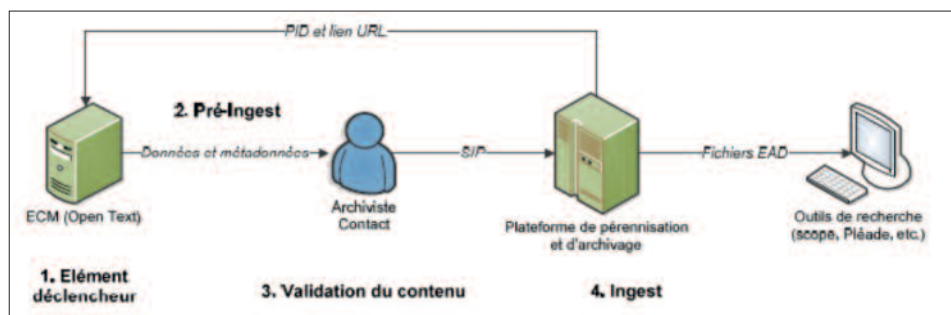
Fig. 3. Modélisation du processus de versement des archives électroniques depuis le système ECM.
