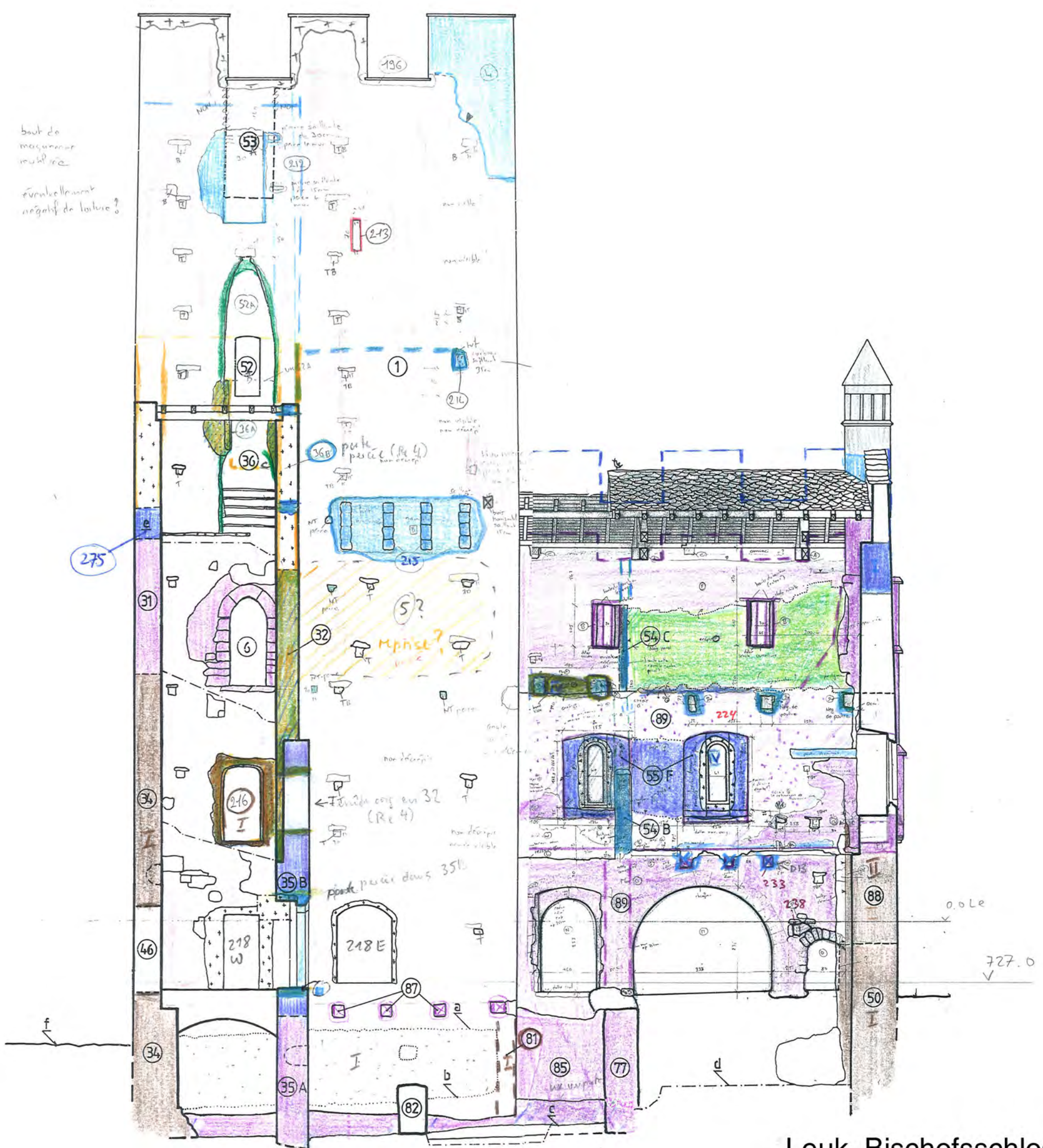
Leuk, Bischofsschloss Turm-Südfassade mit Schnitt durch das Treppenhaus und Nordwand des Palasannexes
