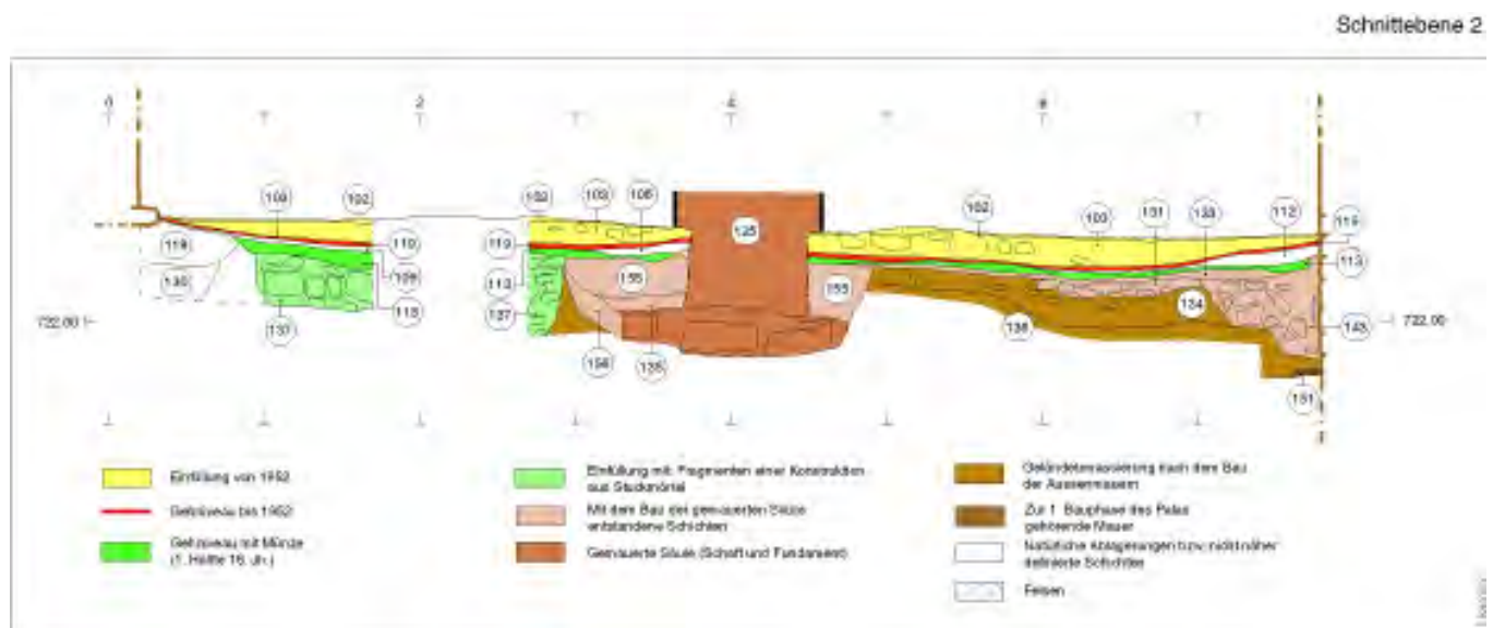
Abb.26 Palas, Keller. Sondierschnitt westlich der gemauerten Säule (Ostprofil). Schematische Darstellung der Erdschichten.
