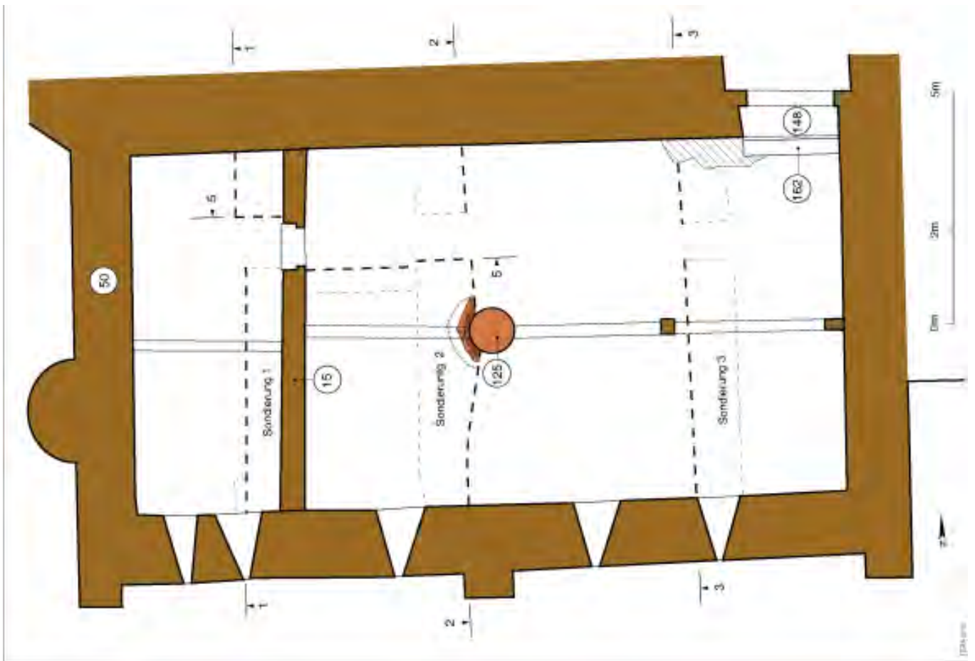
Abb.25 Palas, Keller. Situierung der Sondierungen von 2001.
