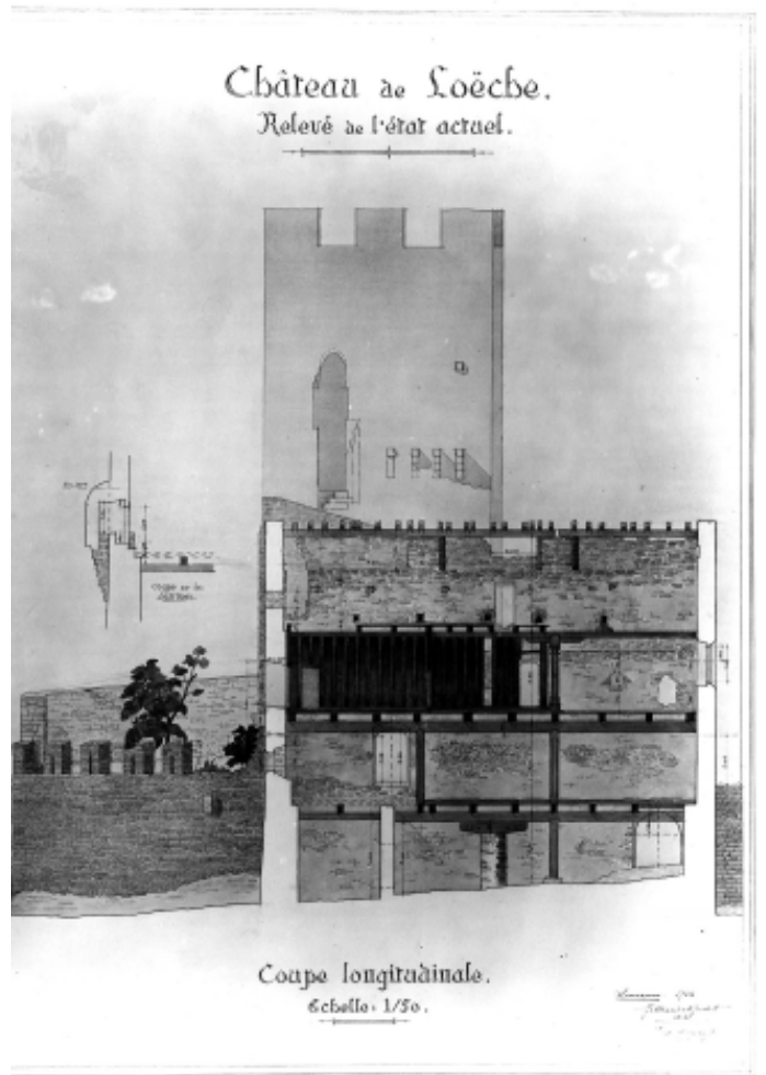
Abb.54 Längsschnitt durch den Palas, gegen Norden. Aufnahmeplan von 1911.
