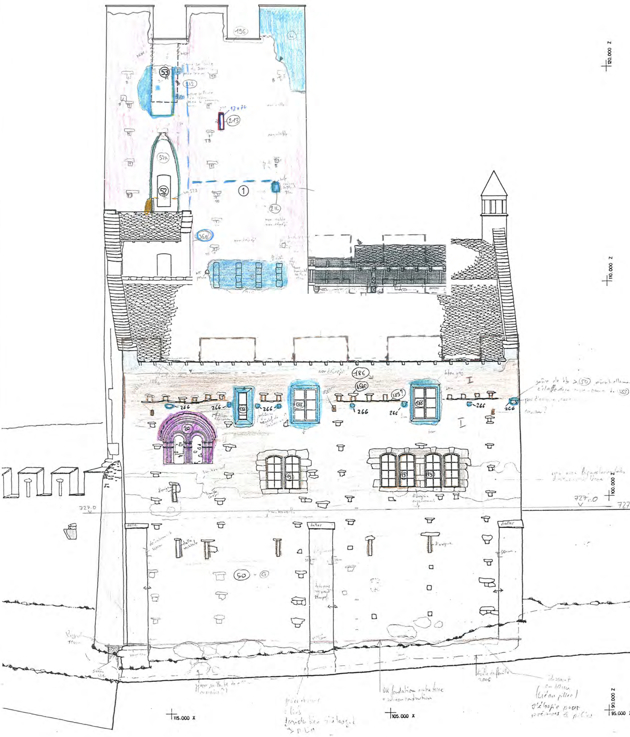
Leuk, Bischofsschloss Palas, Südfassade
