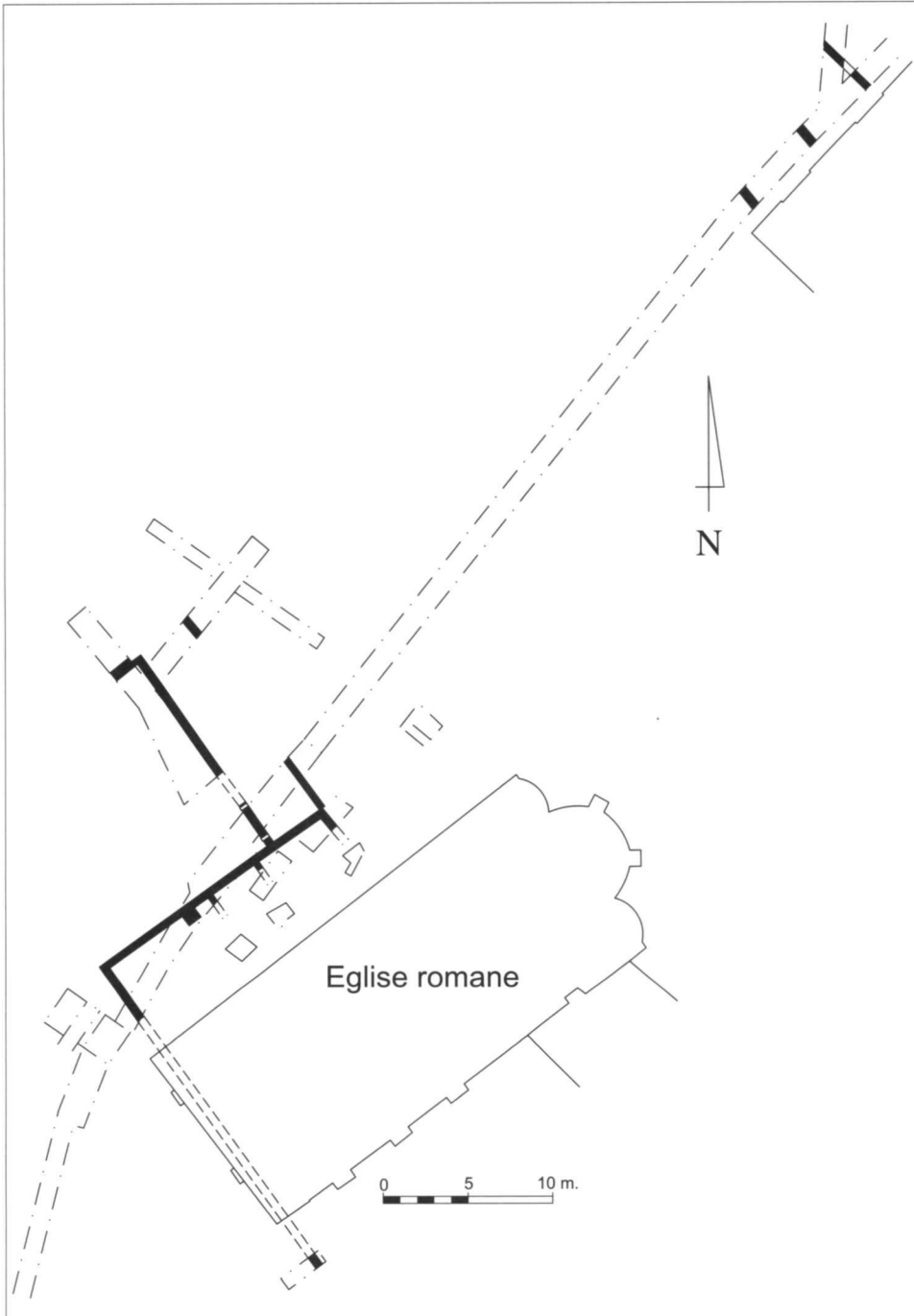
Fig. 2 – Chamoson, Saint-Pierre-de-Clages. Plan d'ensemble des vestiges de l'établissement d'époque romaine repérés au centre du village. Ech. 1 : 400.
