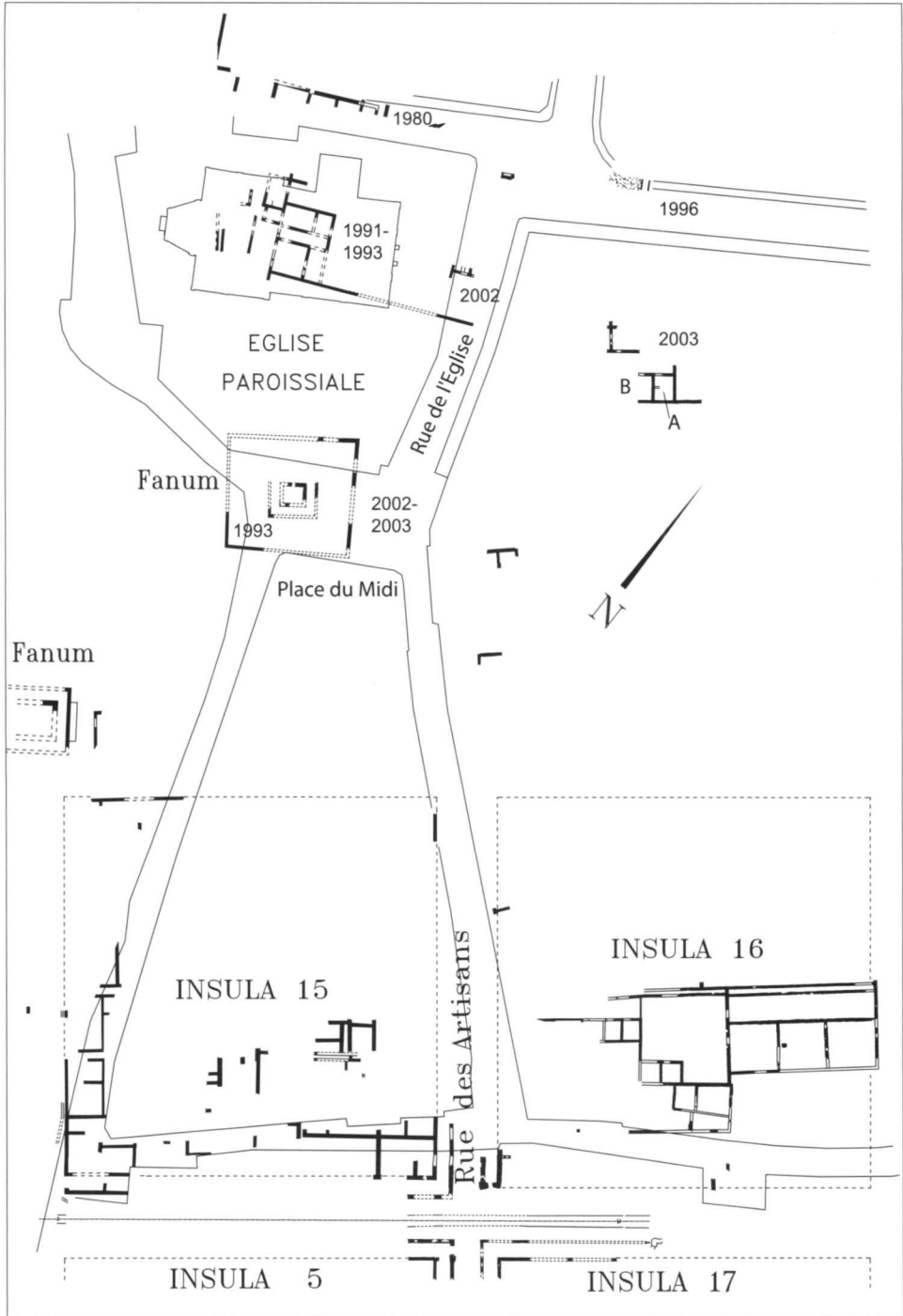
Fig. 6 – Martigny, Quartier du Coin de la Ville et de la Délèze: Plan d'ensemble du dernier état des constructions d'époque romaine. Ech. 1: 1000.
