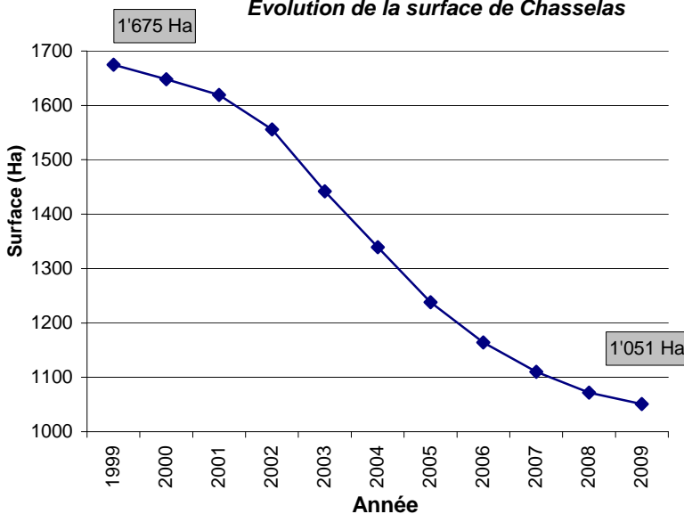
Evolution de la surface de Chasselas
