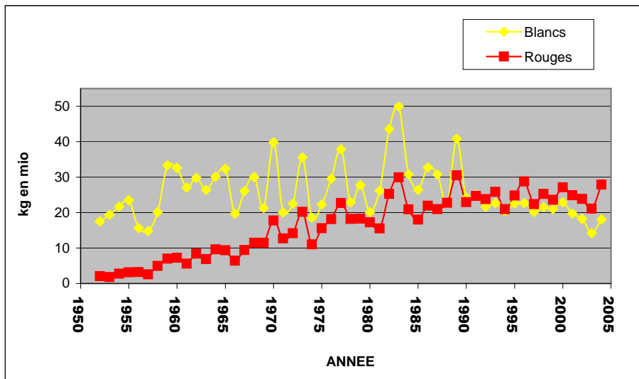
Répartition blanc-rouge 1952-2004
