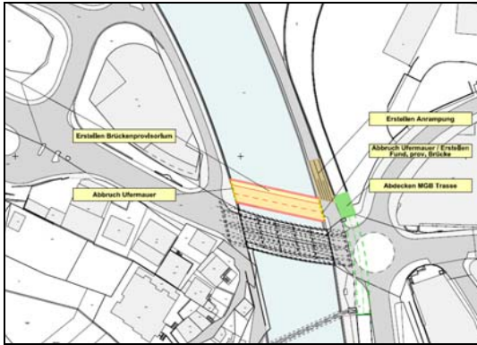
Bauphase: Erstellen der provisorischen Brücke
