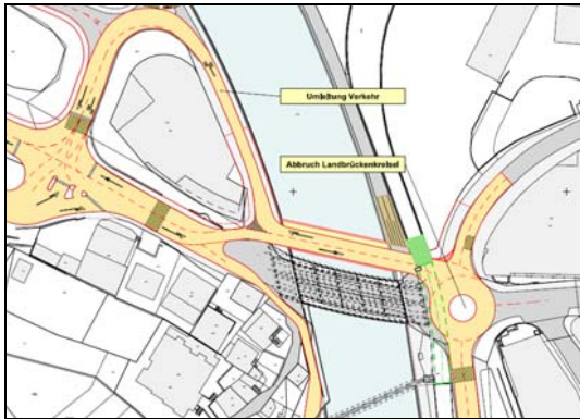
Bauphase: Verkehrsumleitung
